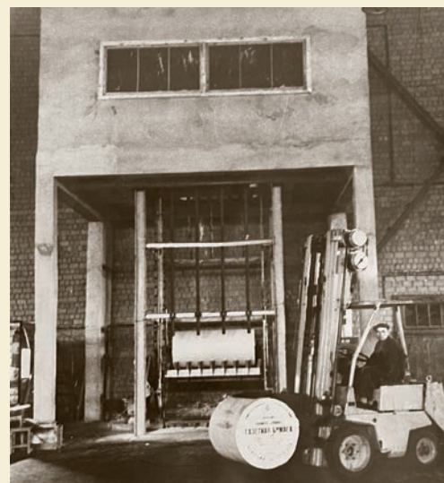
Эlevator для спуска рулонов бумаги на склад готовой продукции.
