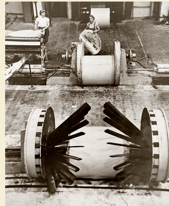
Упаковочный станок бумагоделательной машины №6.
