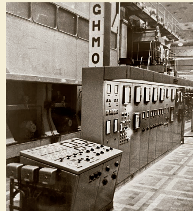
Пульт управления сушильной частью бумагоделательной машины №6.
